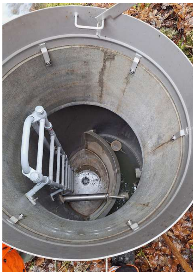
Kontrollschacht direkt vor der Kaltbrunnenquelle und Sicht in die Tiefe
